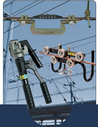
Fahrdraht Werkzeuge
